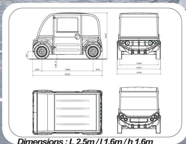
Dimensions : L 2,5m / l 1,6m / h 1,6m
