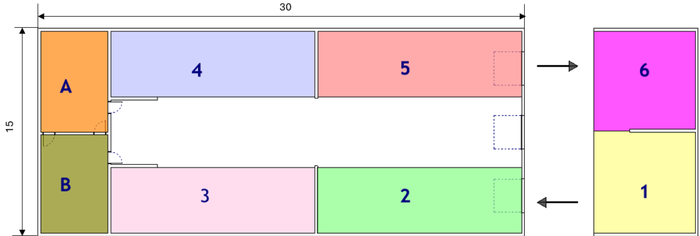
Vue en plan du plateau technique
