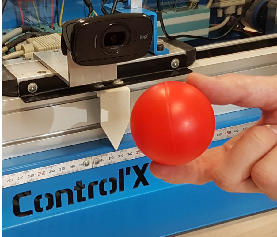
Suivi de cible par analyse d'image sous Simulink
