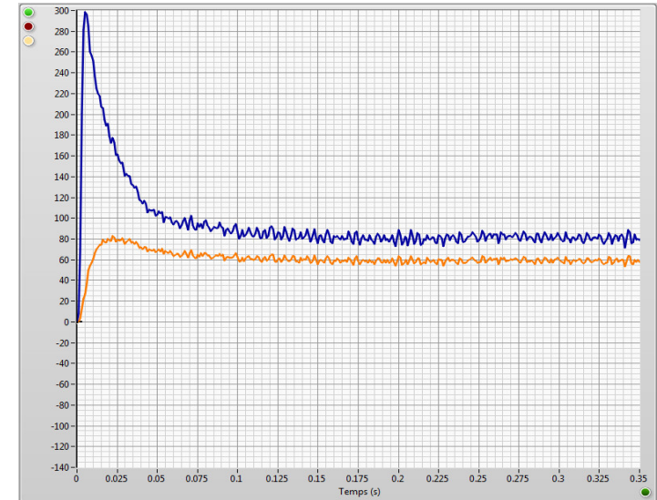
Puissances électrique (W) et mécanique (W) au cours d'un essai de réponse indicielle
