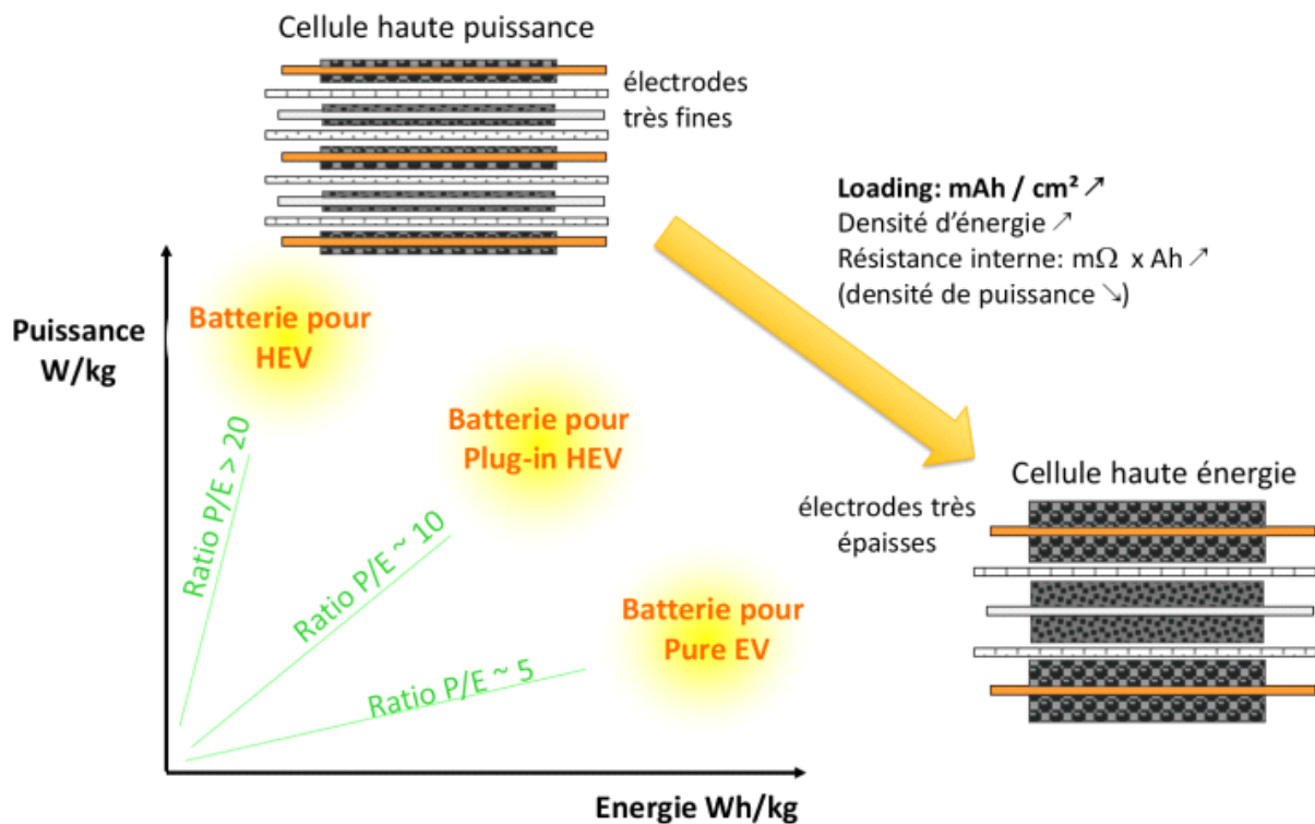
Figure 7 : Cellules Li-Ion typée Energie ou Puissance, source Renault
