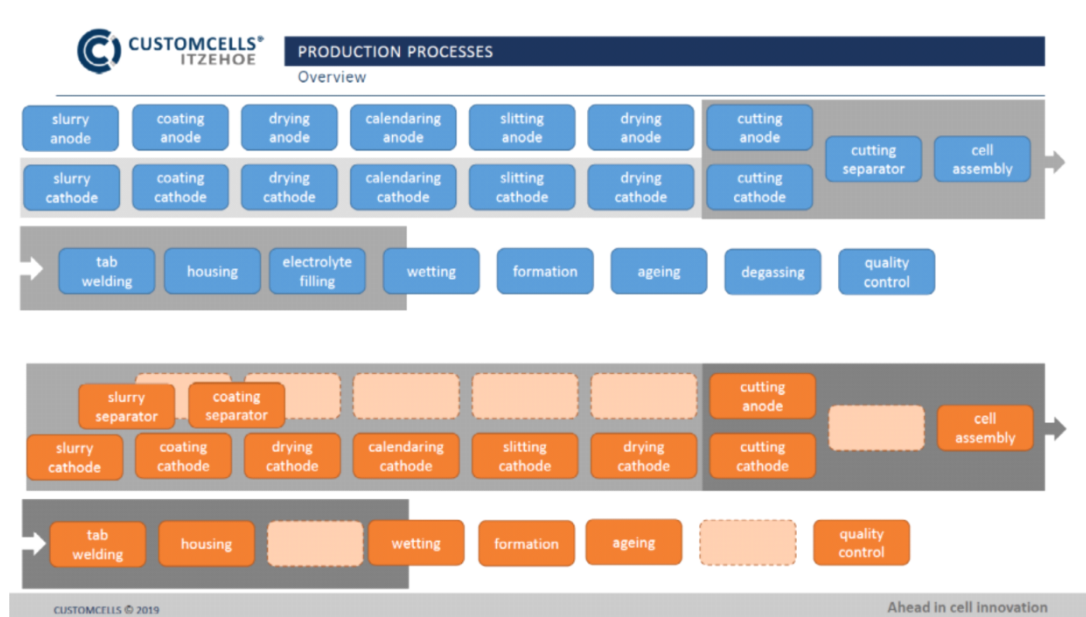
Figure 16 : Comparaison des procédés de prototypage de cellules Li-ion (en haut) et Li tout solide (en bas), source [19]
