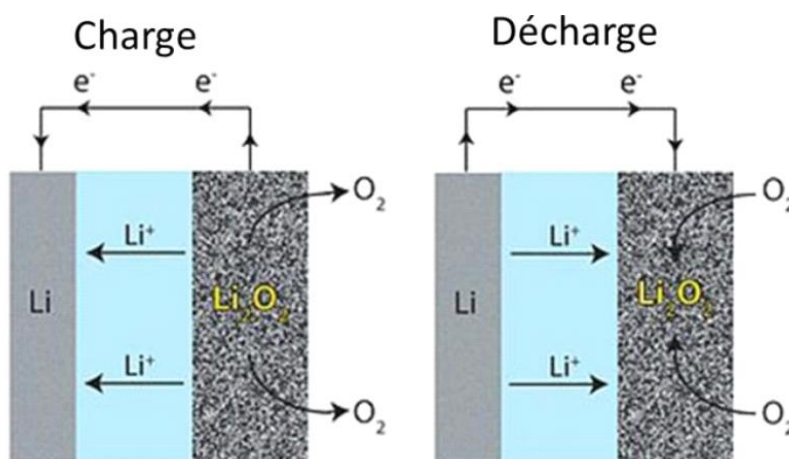
Figure 19 : Principe de fonctionnement d'une batterie Lithium-air, source [21]
