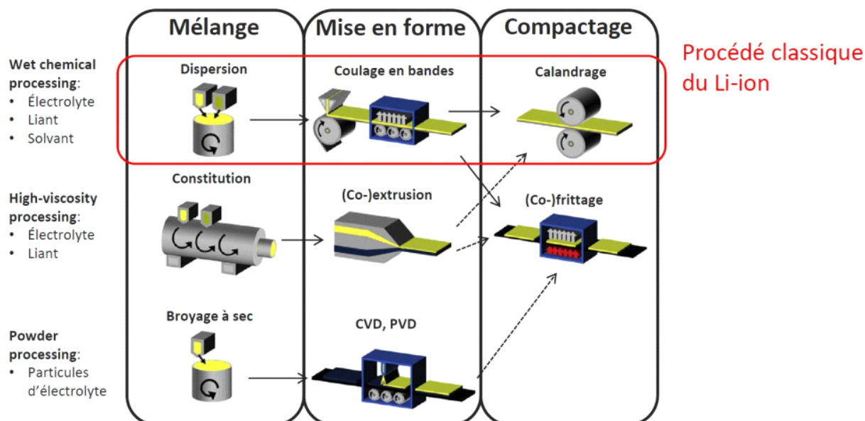
Figure 15 : Fabrication de matériaux de batterie Li tout solide par comparaison au procédé Li-ion, source [18]
