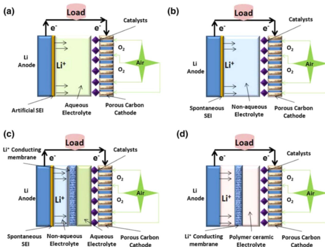
Figure 20 : Différentes configurations de batterie Li-air, source [21]
