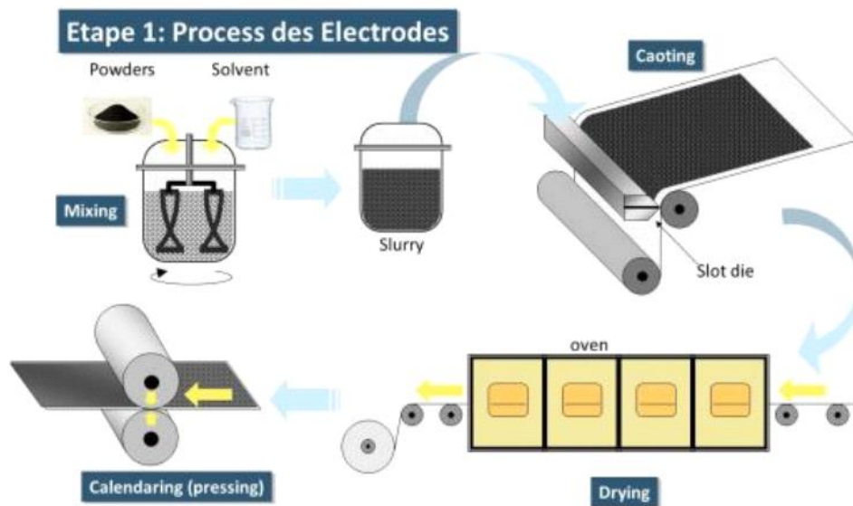
Figure 3 : Process des électrodes, source Renault
