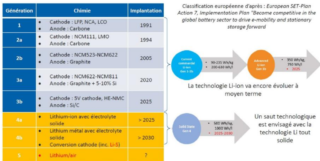
Figure 12 : Feuille de route des technologies de batterie, source [15]
