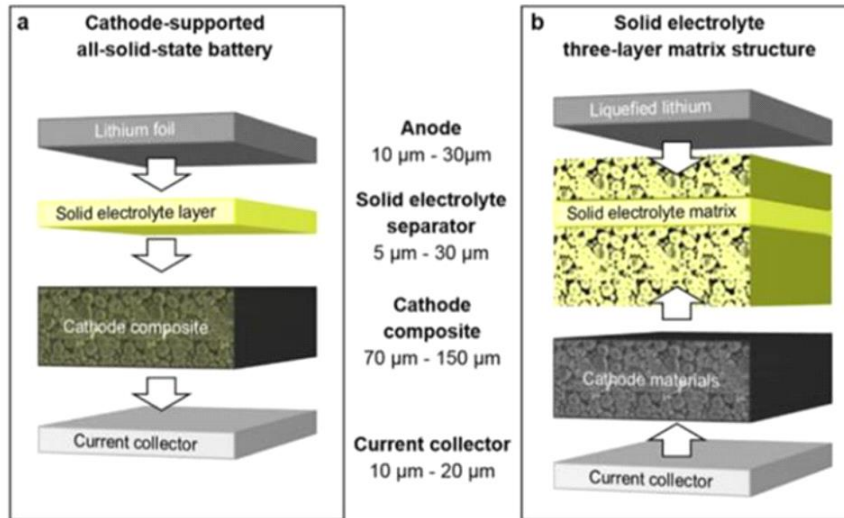
Figure 17 : Variantes de design de cellules Li tout solide, en fonction de la nature des matériaux combinés, source [18]
