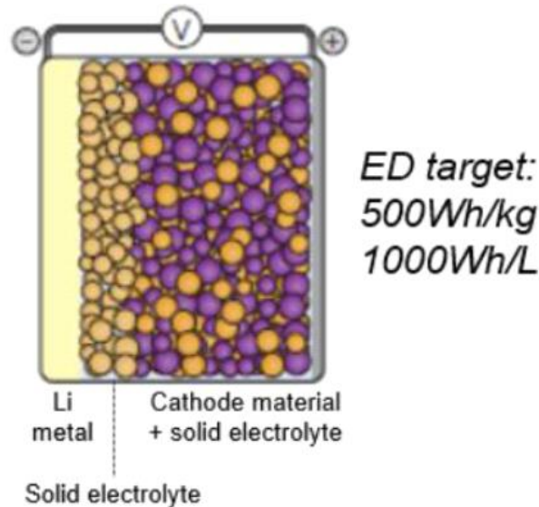
Figure 13 : Représentation schématique d'une cellule de batterie Lithium tout solide, source [16]
