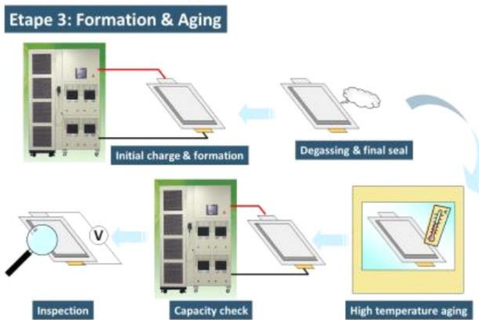
Figure 5 : Formation et vieillissement du module, source Renault
