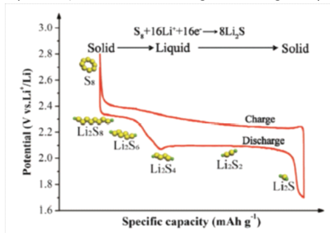
Figure 18 : Profil de charge/décharge de batterie LiS (positive S8), source [20]
