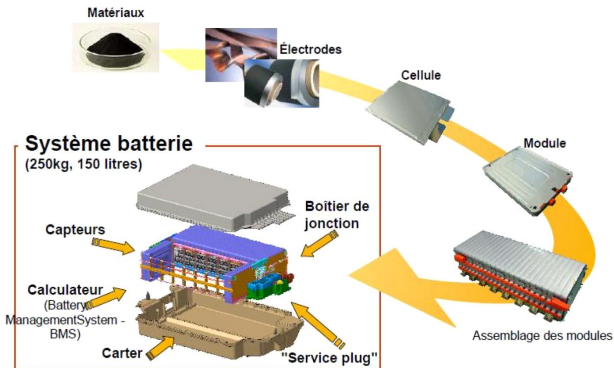
Figure 6 : De la cellule Li-Ion au pack batterie, source Renault
