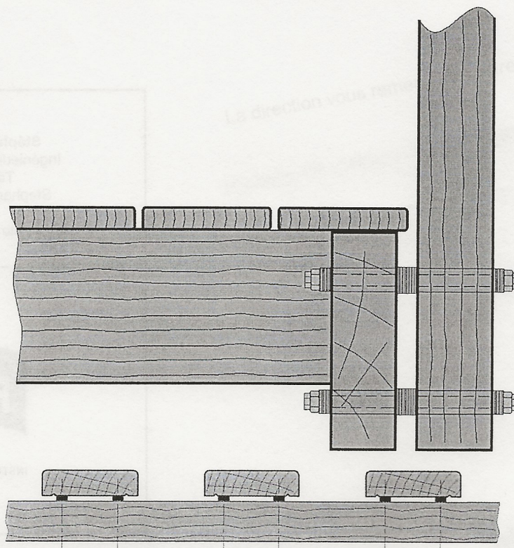
Figure n° 1 : Conception drainante
