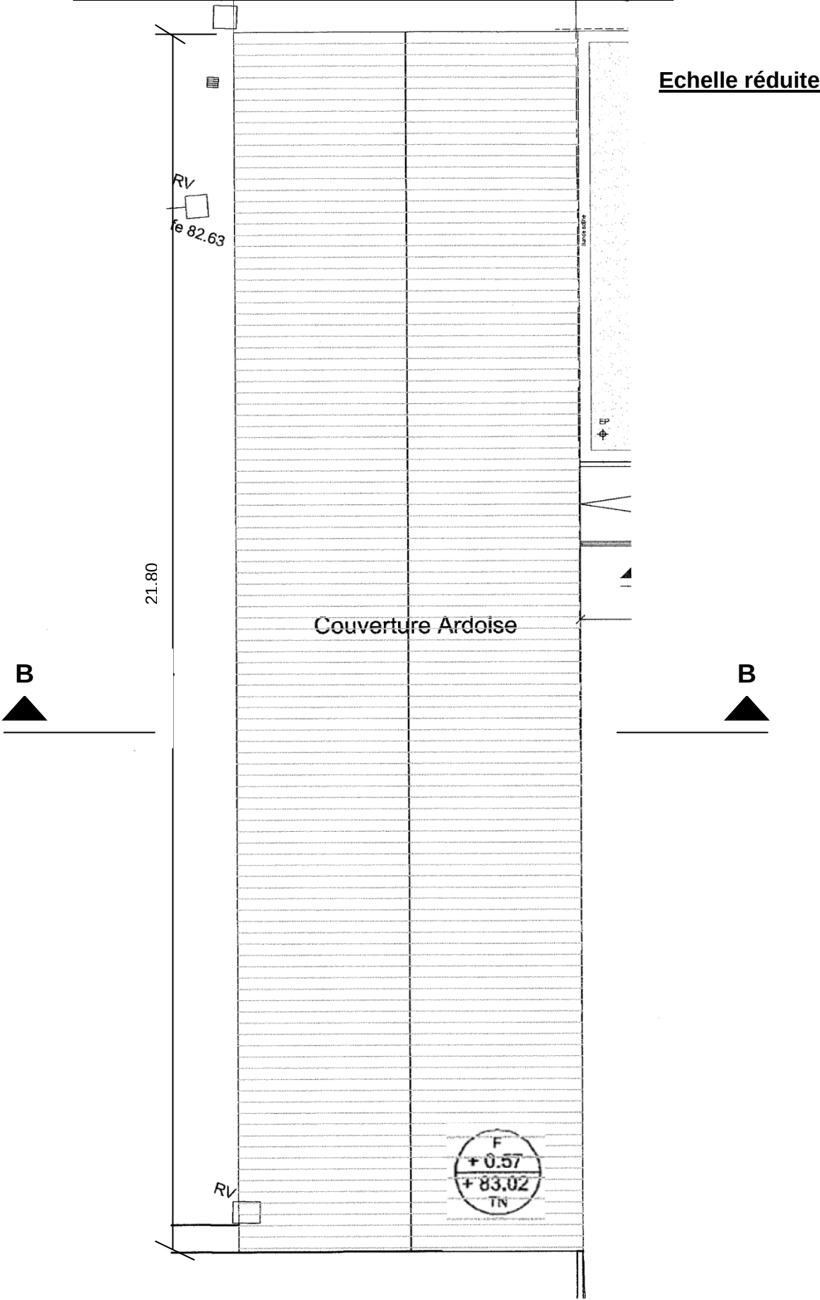
PLAN TOITURE ZONE « PREAU »
