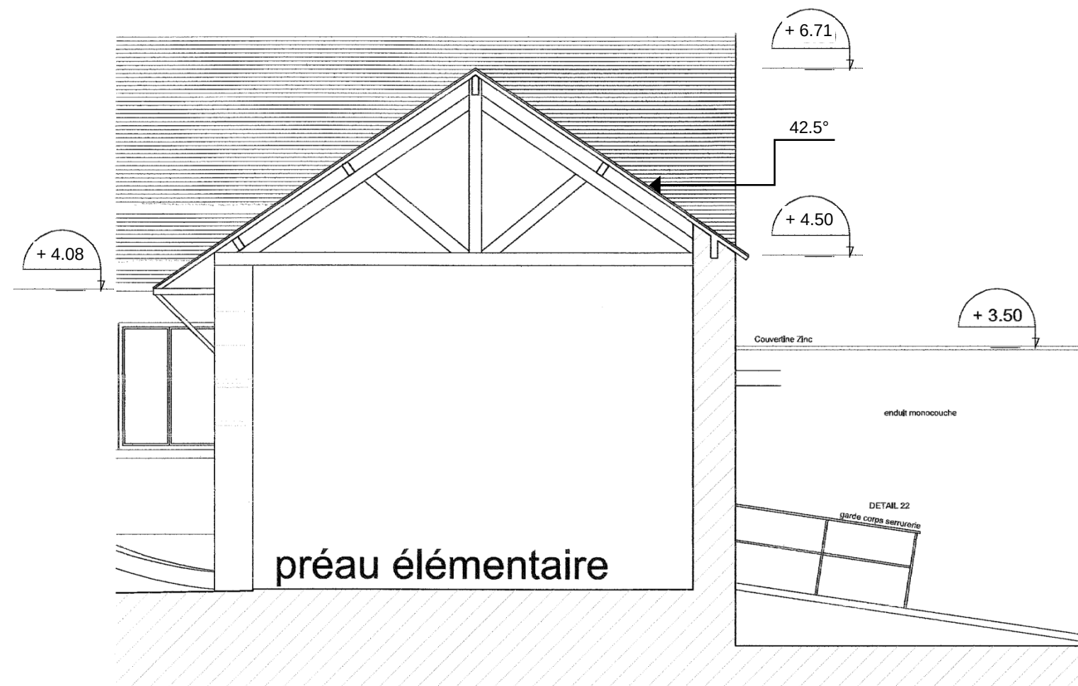
COUPE B.B.
