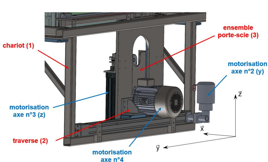
Figure 19 : Vue 3D partielle du module de coupe
