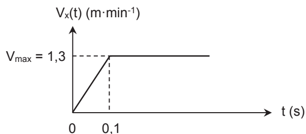
Figure 7 : Loi de vitesse - axe n°1
