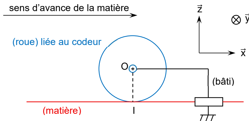
Figure 17 : Schéma cinématique
