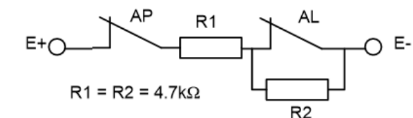
Schéma 1: schéma de principe de raccordement d'un détecteur
