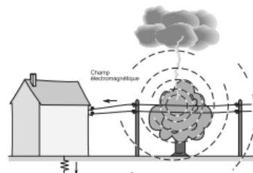
Coup de foudre proche de bâtiments (surtension due au rayonnement électromagnétique).
