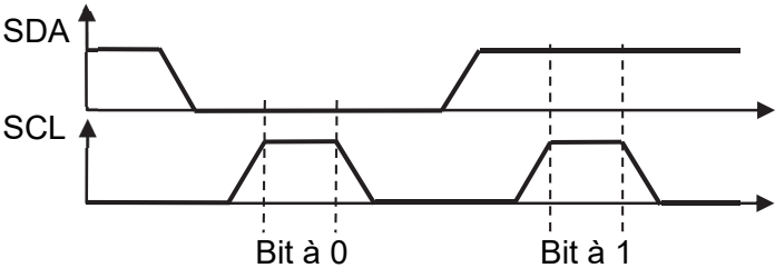
Figure 11 : exemple de signaux SDA et SCL
