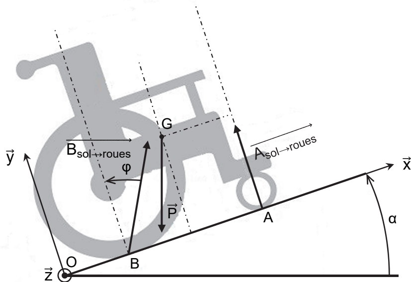
Figure 8 : modélisation des actions mécaniques extérieures exercées sur le fauteuil roulant
