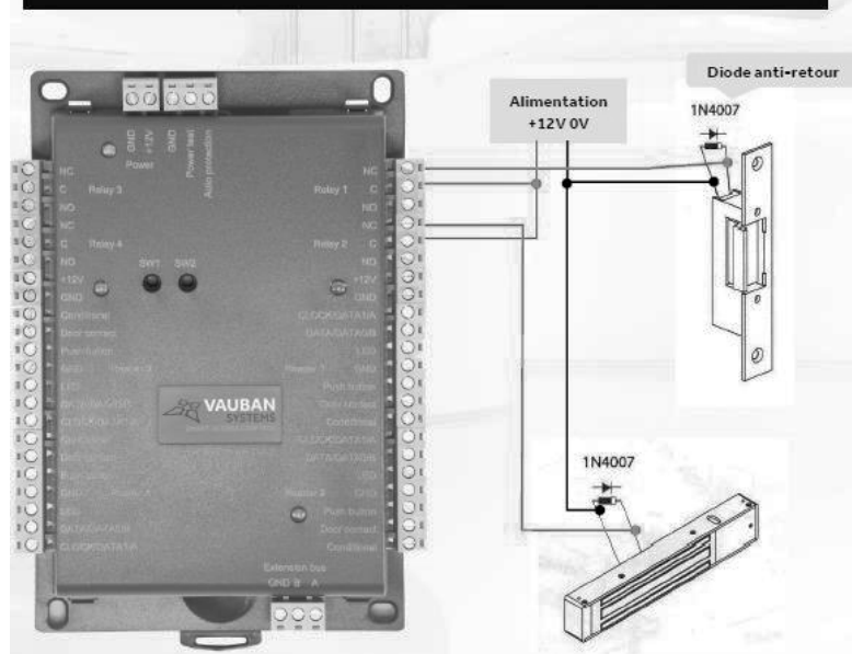
Exemple de raccordement
