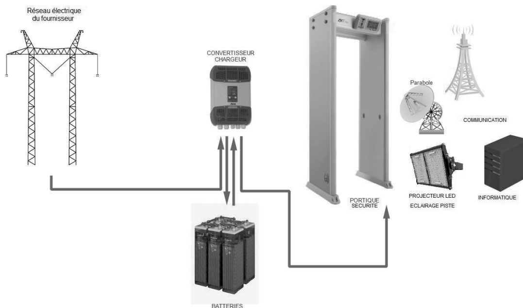
Schéma 2. Synoptique alimentation électrique aérodrome
